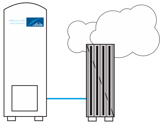
Suskystinto deguonies išsiplečimas. 1 litras suskystinto deguonies sudaro 860 litrų dujinio deguonies.
